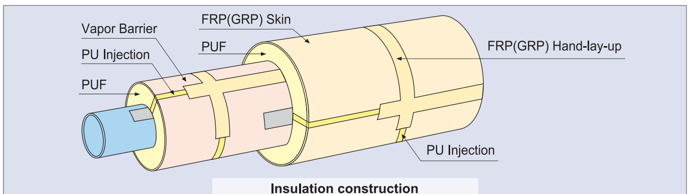
Moss type LNG carrier pipe insulation
